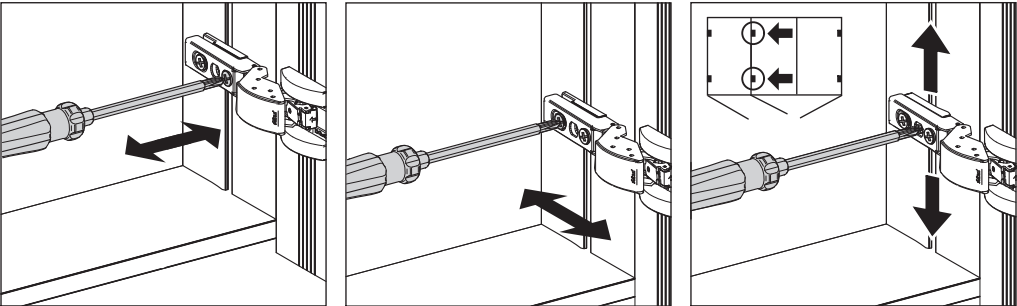
Seitenverstellung - Réglage latéral - Lateral setting Tiefenverstellung - Réglage profondeur - Depth adjustment Höhenverstellung - Réglage hauteur - Height adjustment
