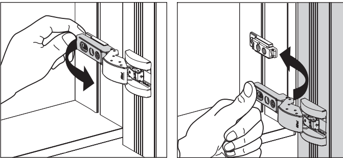
Demontage - Démontage - Disassembly Montage - Assemblage - Assembling
