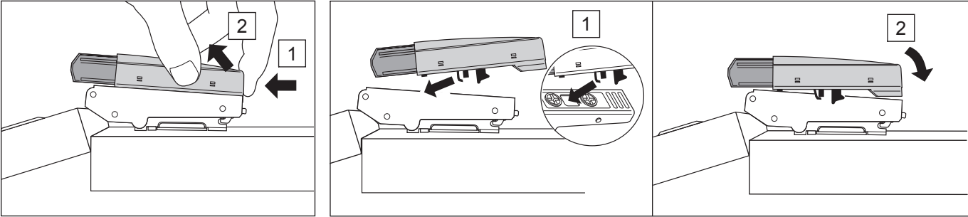
Demontage - Démontage - Disassembly Montage - Assemblage - Assembling
