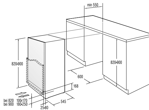
RBIU / RIU / FIU 6092 AW
