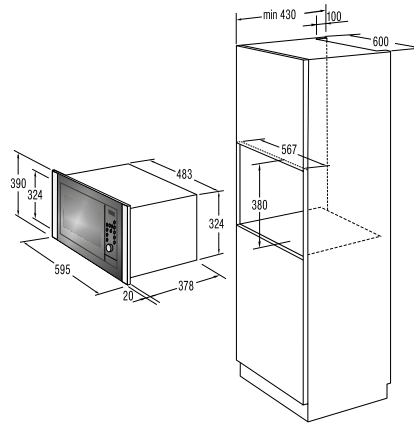
BM 6340 AX / BM 5240 AX BM 1240 AX
