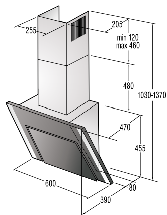
DVG 6640 X / DVG 6640 W
