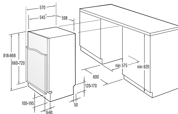
GV 64325 XV / GV 62324 / GV 61224
