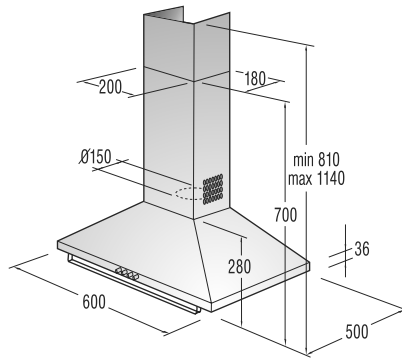
DK 63 CLI / CLB
