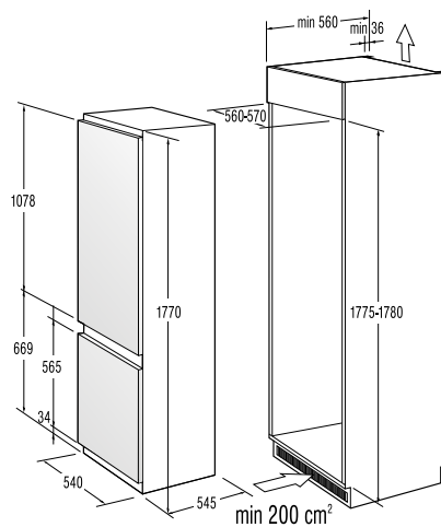
RKI 4182 EW / RKI 4181 AW
