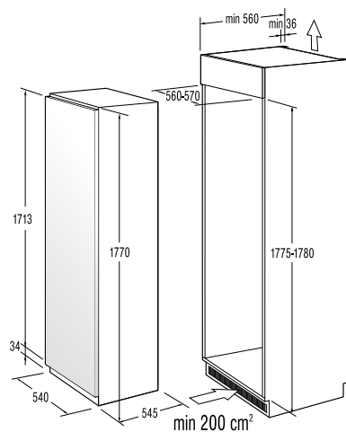
RBI 4182 BW / RI 4182 AW
