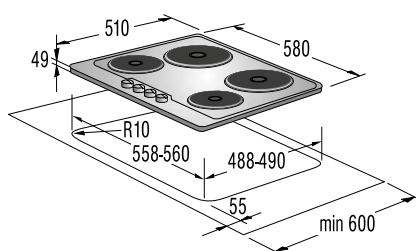
E 6N1 AX
