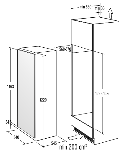
RBI 4122 AW / RI 4122 AW
