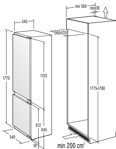
RKI 5182 EW / RKI 5181 AW
