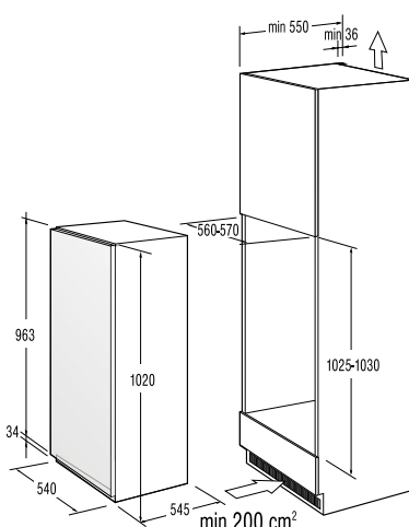
RBI 4102 AW / RI 4102 AW
