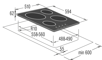
ECK 63 CLI / CLB
