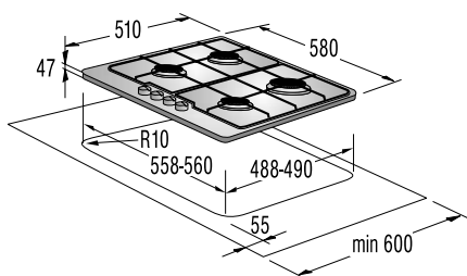
GW 6N41 IX / G 6N40 IX
