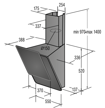
DKG 552 ORA-S / DKG 552 ORA-W
