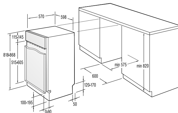
GI 63324 X / GI 61224 X/W
