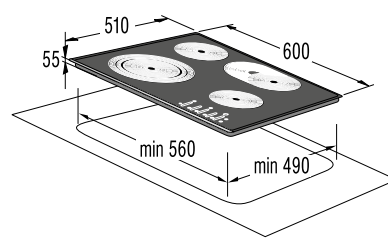
ECT 680 ORA / ECT 680 ORA-W
