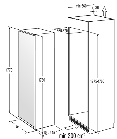
RBI 5182 BW / RI 5182 AW
