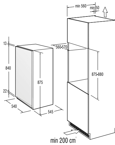
RBI 4093 AW / RBI 4092 AW / RI 4092 AW
