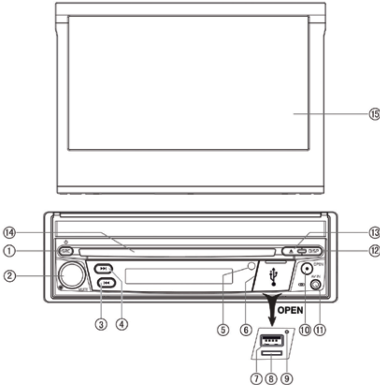
Commandes et voyants du MAC 410
