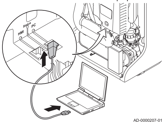
Abb.33 Anschließen eines PCs/Laptops
