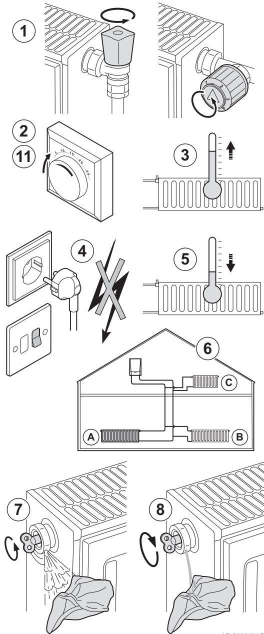
Abb.61 Entlüften der Anlage
