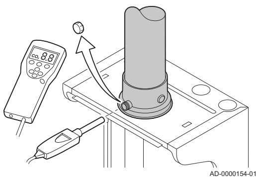
Abb.42 Prüföffnung für Abgas
