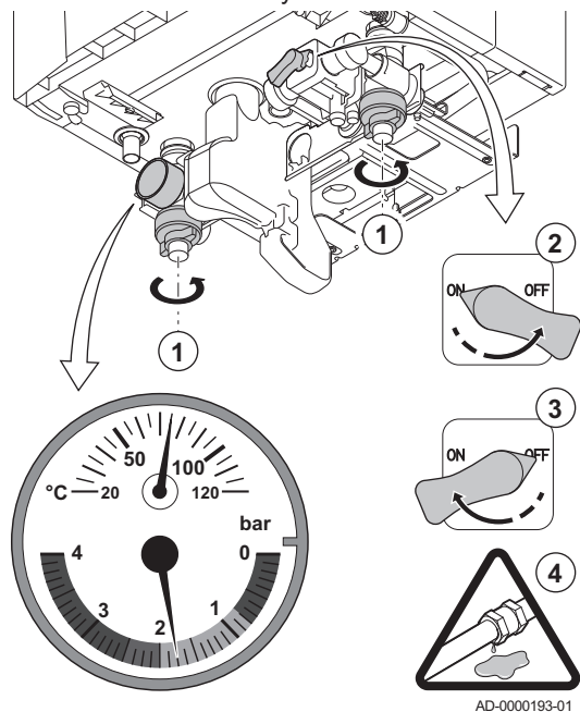
Abb.38 Befüllen des Systems
