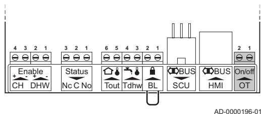
Abb.27 Anschluss des Frostschutzthermostats
