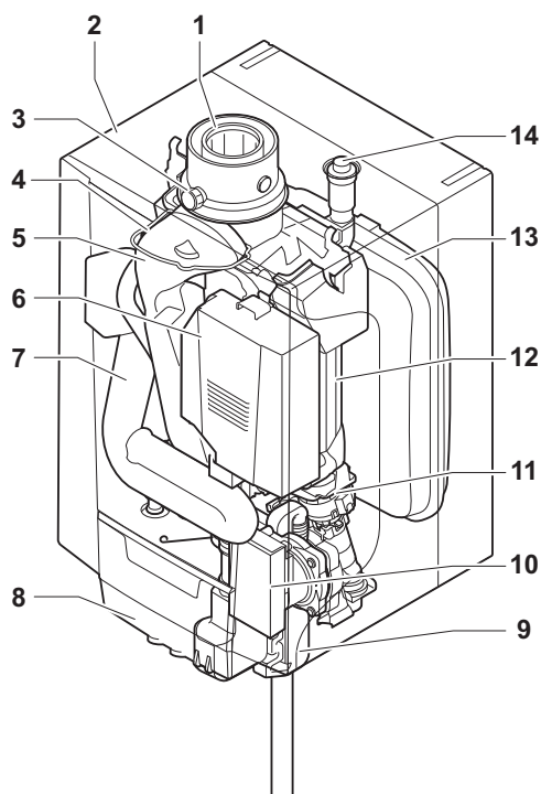
Abb.8 Hauptbestandteile Tzerra M28C -
