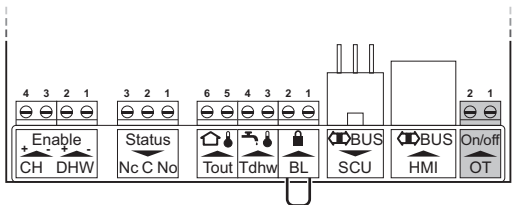
Abb.24 Anschluss des Ein/Aus-Thermostats
