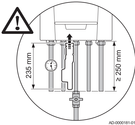
Abb.14 Platz für Einbauten unter dem Kessel
