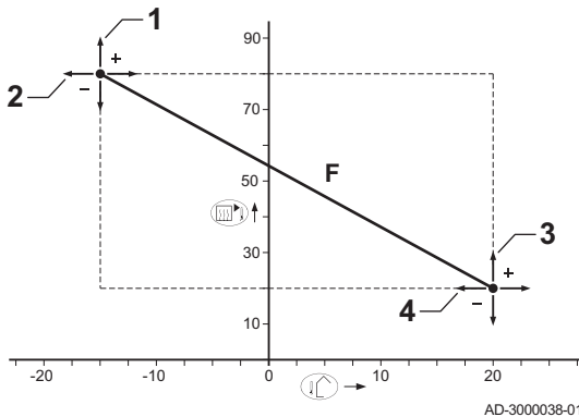
Abb.26 Heizkennlinie
