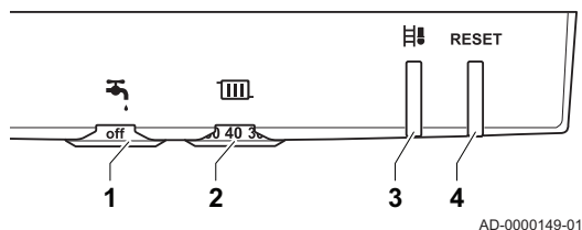
Abb.62 Kesselschaltfeld
