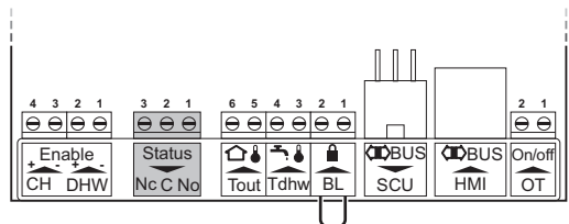
Abb.30 Betriebssignal und Fehlersignal
