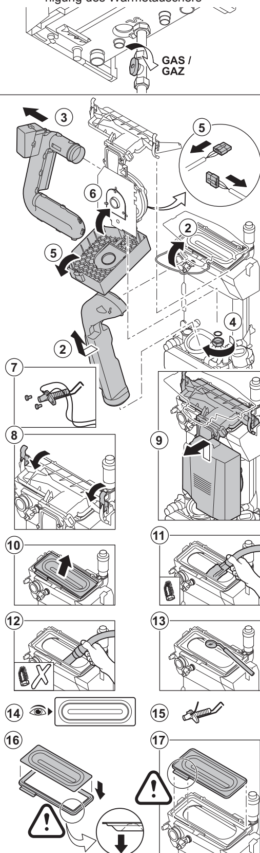
Abb.54 Überprüfung des Brenners und Reinigung des Wärmetauschers
