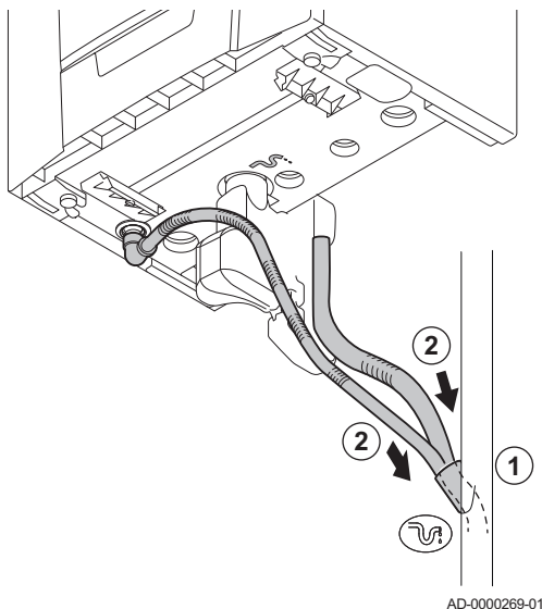
Abb.18 Anschluss der Kondensatablaufleitung
