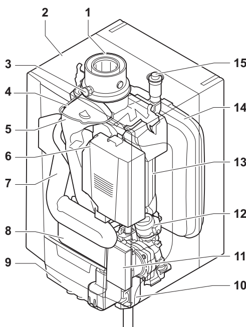
Abb.8 Hauptbestandteile Tzerra M28C -
