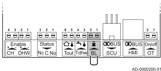
Abb.32 Sperreingang
