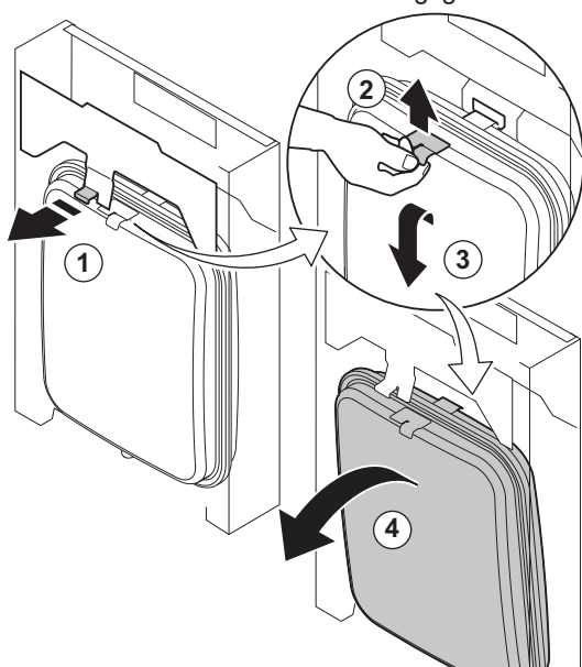
Abb.60 Entfernen des Ausdehnungsgefäßes
