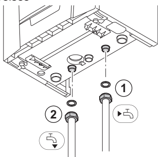
Abb.17 Anschließen des sekundären Heizkreises
