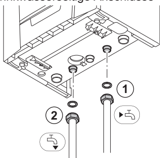
Abb.16 Trinkwasserseitige Anschlüsse
