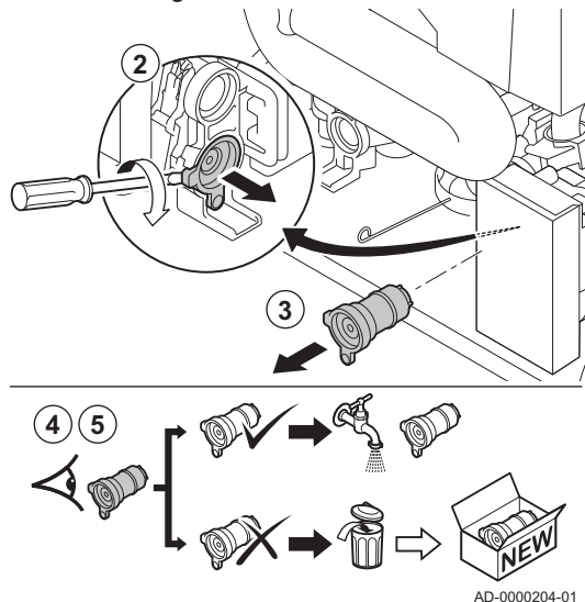
Abb.58 Reinigen des Wasserfilters
