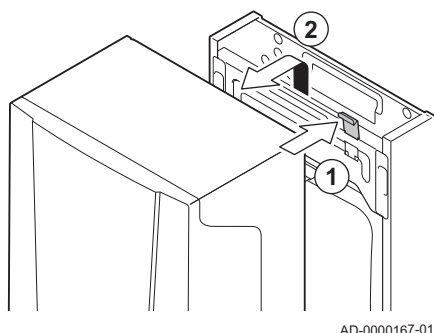
Abb.59 Entfernen des vorderen Teils des Kessels
