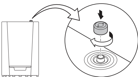
Abb.19 Automatischer Schnellentlüfter
