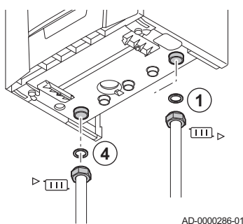
Abb.15 Anschluss des Heizkreises
