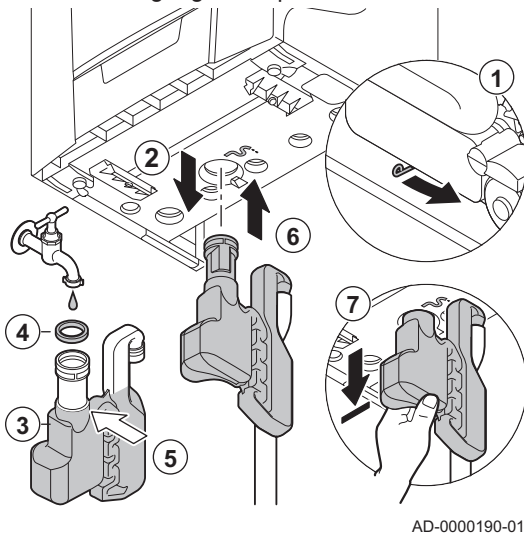
Abb.53 Reinigung des Siphons
