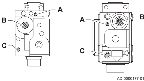
Abb.39 Prüföffnungen der Gasventilbaugruppe
