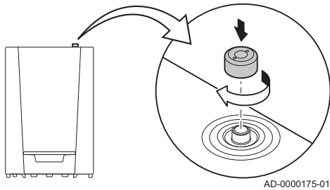
Abb.52 Überprüfung des automatischen Schnellentlüfters
