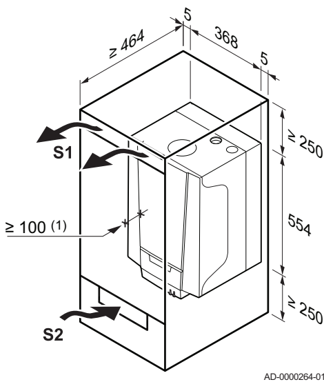
Abb.12 Platz für Belüftung
