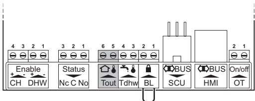
Abb.25 Anschluss eines Außenfühlers
