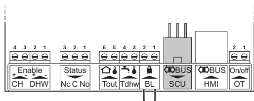
Abb.35 Anschlüsse für optionale Leiterplatten
