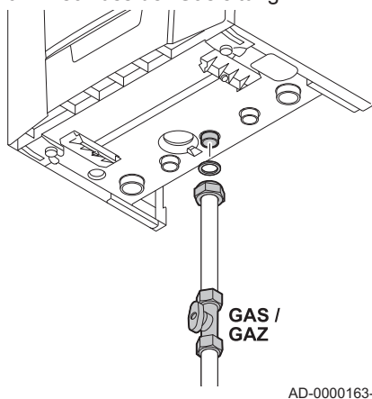
Abb.20 Anschluss der Gasleitung
