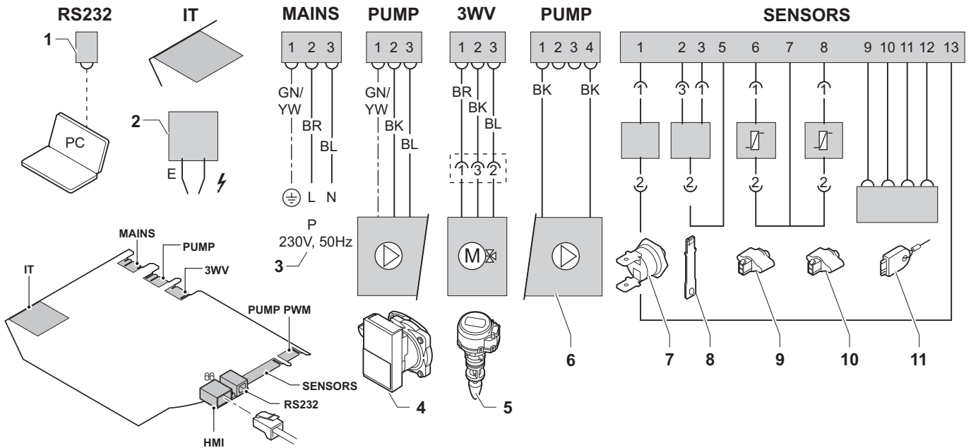
Abb.2 Elektrischer Schaltplan
