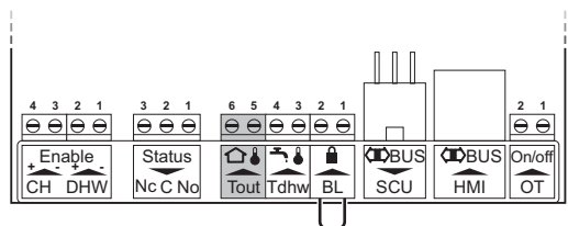
Abb.28 Anschluss eines Außenfühlers
