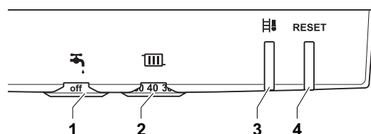
Abb.9 Kesselschaltfeld
