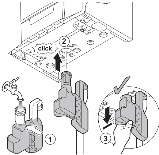
Abb.36 Befüllen des Siphons
