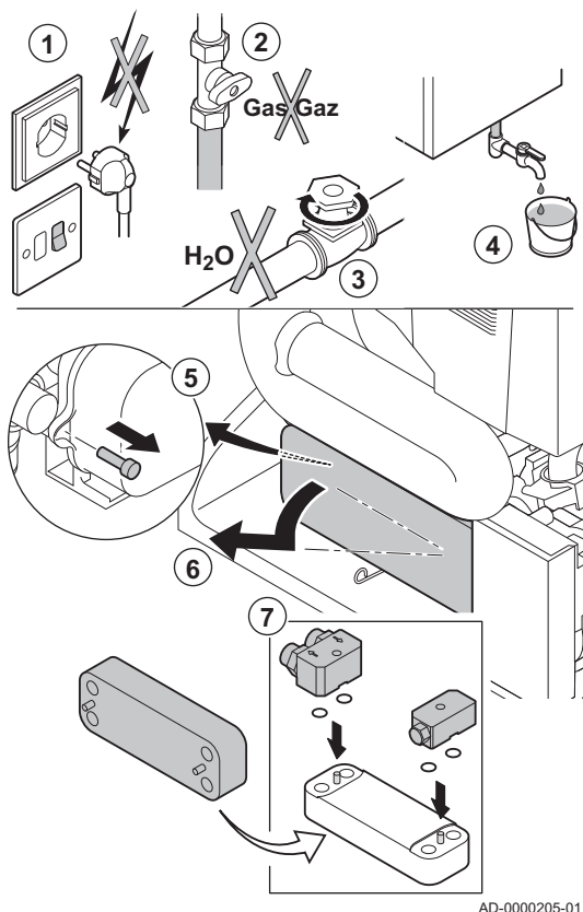
Abb.57 Reinigen des Plattenwärmetauschers
