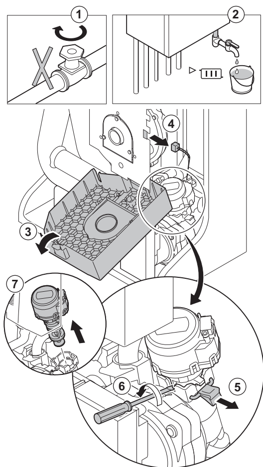
Abb.56 Auswechseln des Dreiwegeventils
