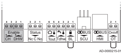
Abb.31 Anschließen des Ein/Aus-Kontakts (Aktivieren)
