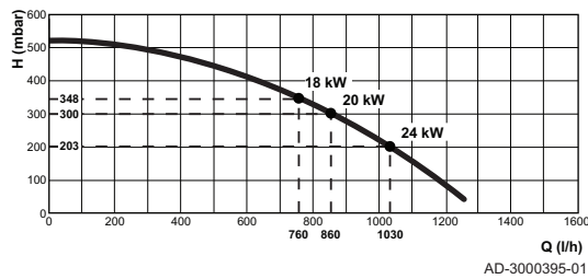
Abb.4 Verfügbare manometrische Höhe Tzerra M -28C
