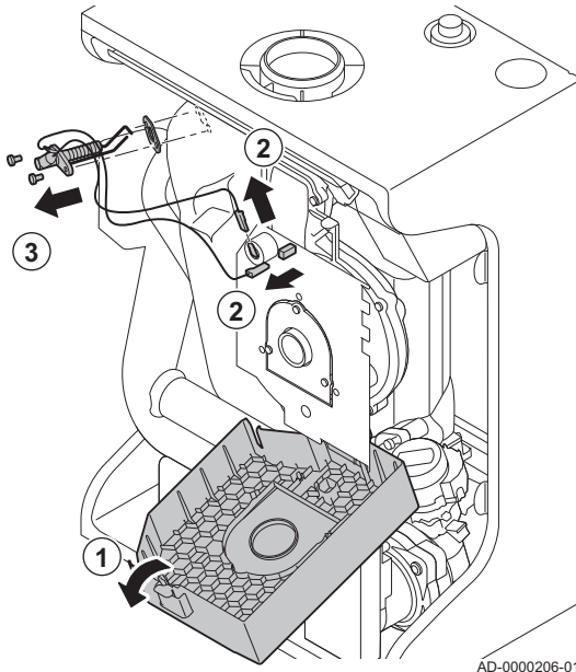
Abb.55 Austausch der Ionisations- bzw. Zündelektrode
