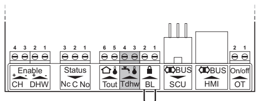
Abb.29 Anschließen des Fühlers/Thermostats für den Warmwasserbereiter
