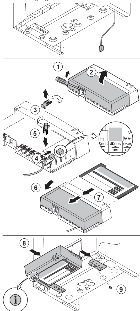
Abb.22 Zugang zu den Anschlüssen
