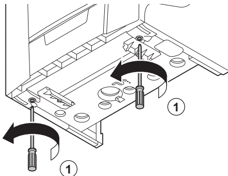
Abb.49 Öffnen des Kessels
