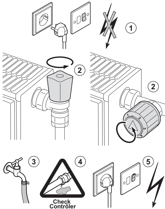
Abb.37 Befüllen des Systems
