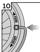
Drahthebel einsetzen von beiden Seiten des Mahlwerks
