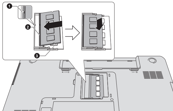
Abbildung 4-9 Speichermodul einsetzen
