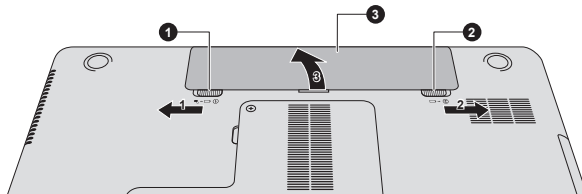
Abbildung 4-5 Akku entsichern -1
