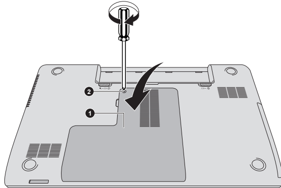
Abbildung 4-10 Speichermodulabdeckung einsetzen
