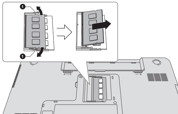
Abbildung 4-11 Speichermodul entfernen
