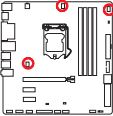
Connecteurs pour ventilateurs en mode tension
