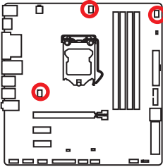
Lüfteranschluss des Spannung-Modus
